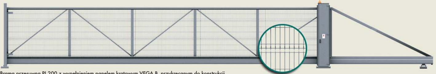
Brama przesuwna PI 200 z wypełnieniem panelem kratowym VEGA B, przykręcanym do konstrukcji - widok od strony posesji
